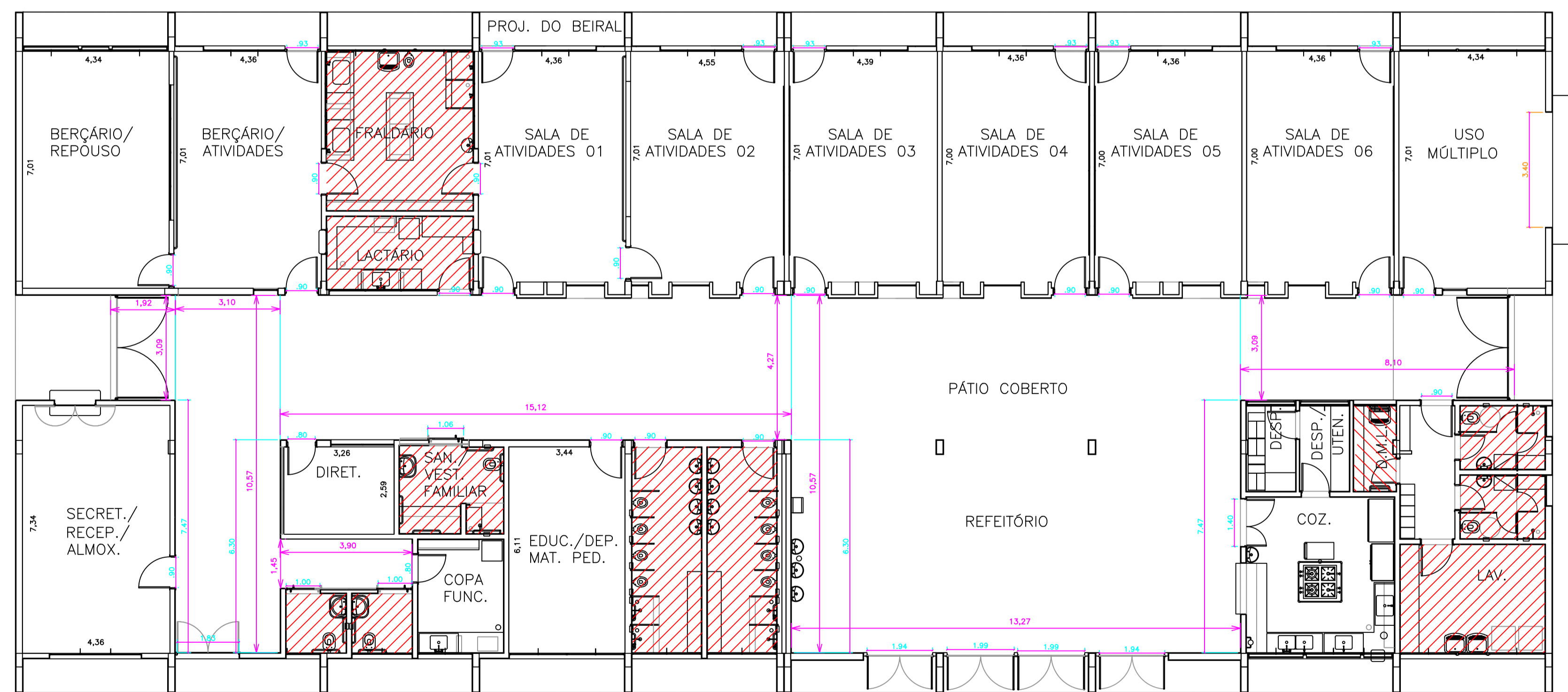
PLANTA BAIXA ESCALA 1:100
